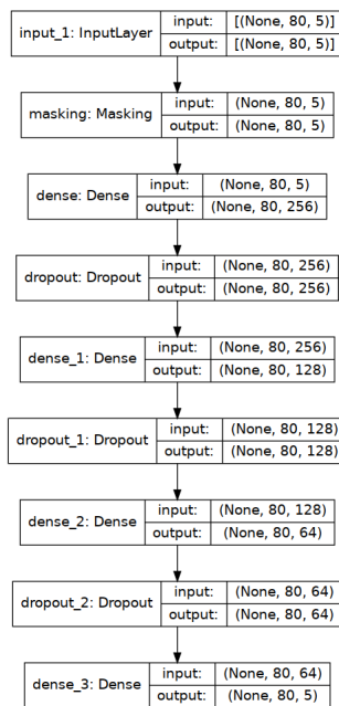
Figura 5.2: Arquitectura de la red neuronal
